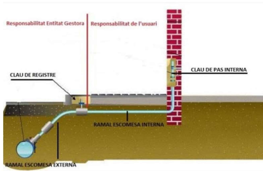
Imatge 1 Esquema de les parts de l'escomesa
