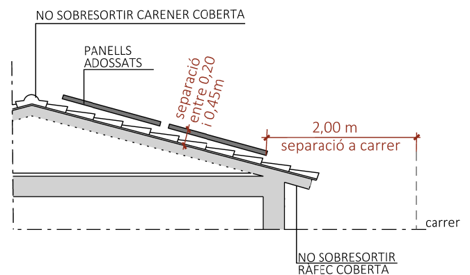
CROQUIS 2 - SECCIÓ COBERTA INCLINADA
