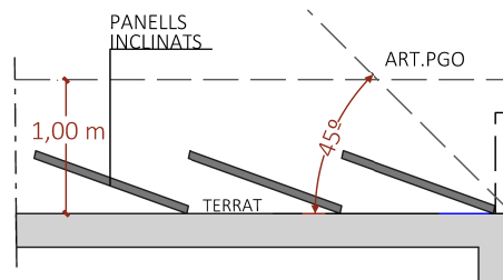
CROQUIS 3 - SECCIÓ COBERTA PLANA
